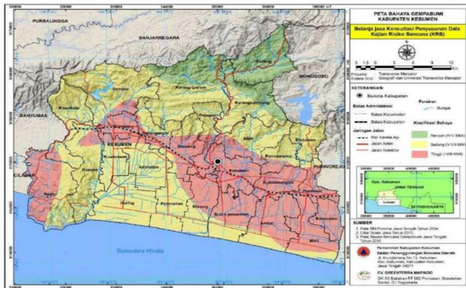
Gambar 2.6 Peta Bahaya Gempa Bumi Kabupaten Kebumen
