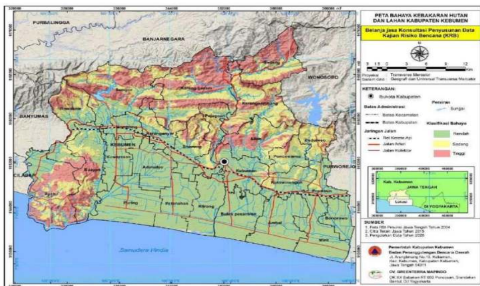
Gambar 2.5 Peta Bahaya Karhutla Kabupaten Kebumen
