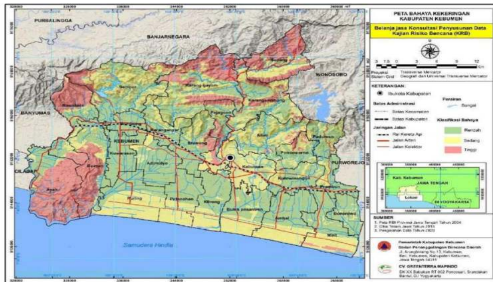
Gambar 2.4 Peta Bahaya Kekeringan Kabupaten Kebumen
