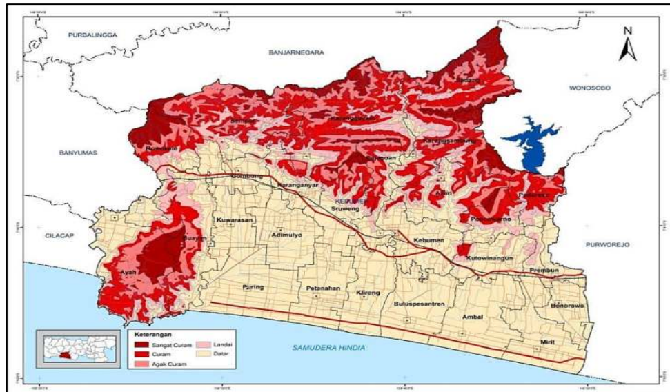
Gambar 2.2 Peta Topografi Kabupaten Kebumen
