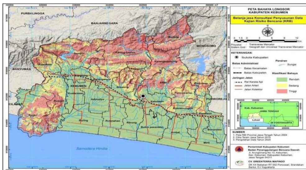
Gambar 2.7 Peta Bahaya Tanah Longsor Kabupaten Kebumen
