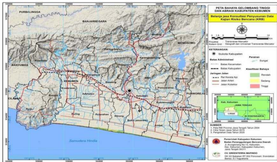
Gambar 2.8 Peta Bahaya Gelombang Ekstrem dan Abrasi Kabupaten Kebumen
